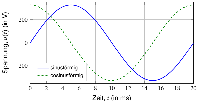
Abbildung: Harmonischer Zeitverlauf einer Spannung mit einer Frequenz von 50 Hz und einem Effektivwert von 230 V
